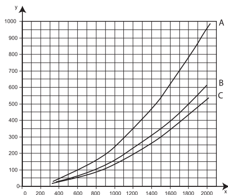
X: debiet, m 3 /u, Y: statische druk, Pa A: Verlengarm 40° gebogen (tot het maximum). B: Verlengarm 90° gebogen. C: Rechte verlengarm.
