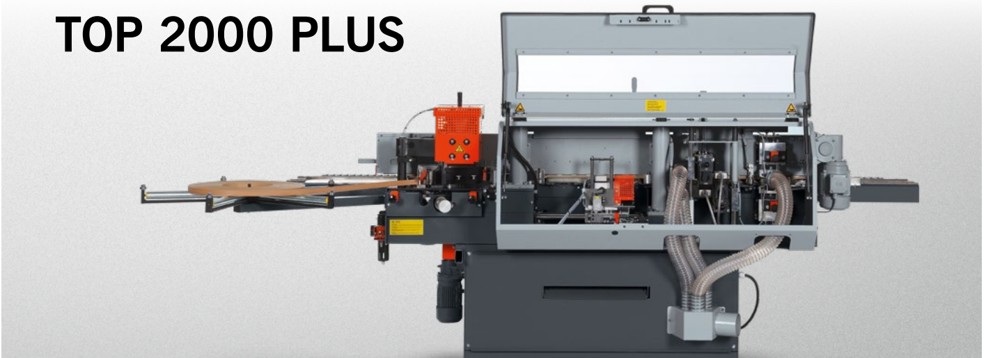
Abbildung zeigt die optionale Ausstattung mit Flächenziehklinge.
